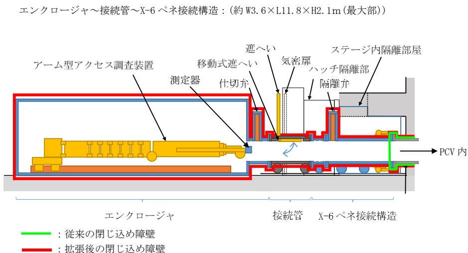
図3 X-6 ペネ エンクロージャ等 構造概略図※
