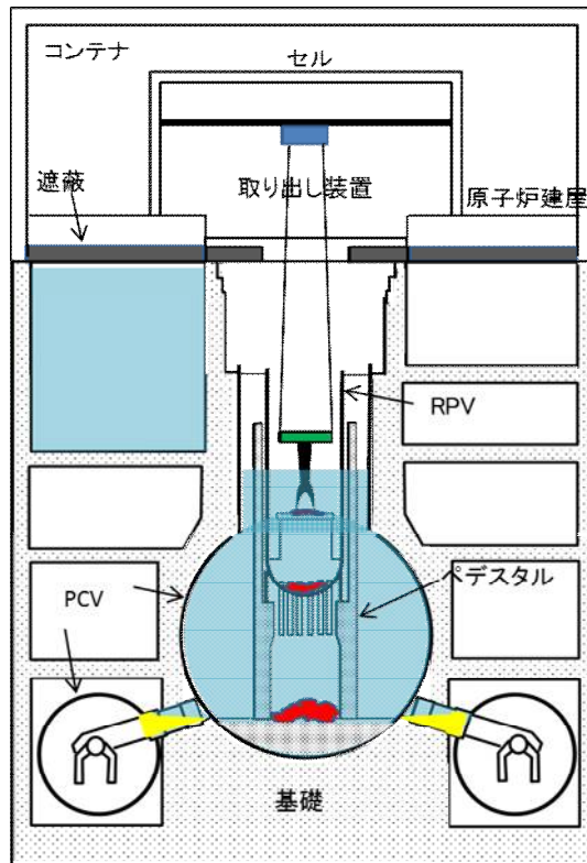
a. 冠水-上アクセス工法
