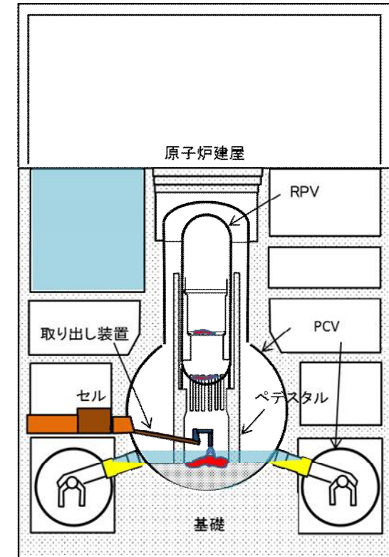
c. 気中-横アクセス工法
