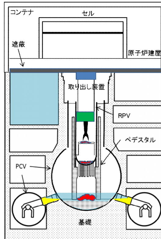
b. 気中-上アクセス工法
